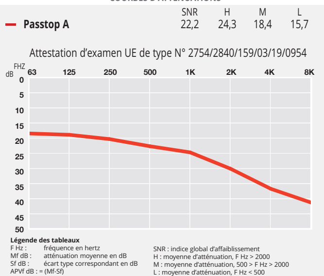
COURBES D'ATTENUATIONS
